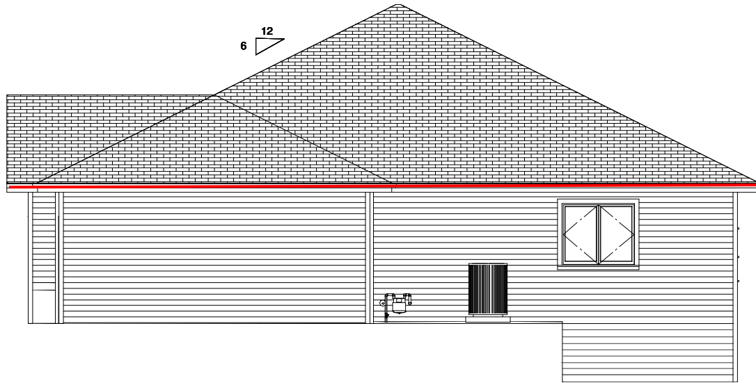
RIGHT ELEVATION
